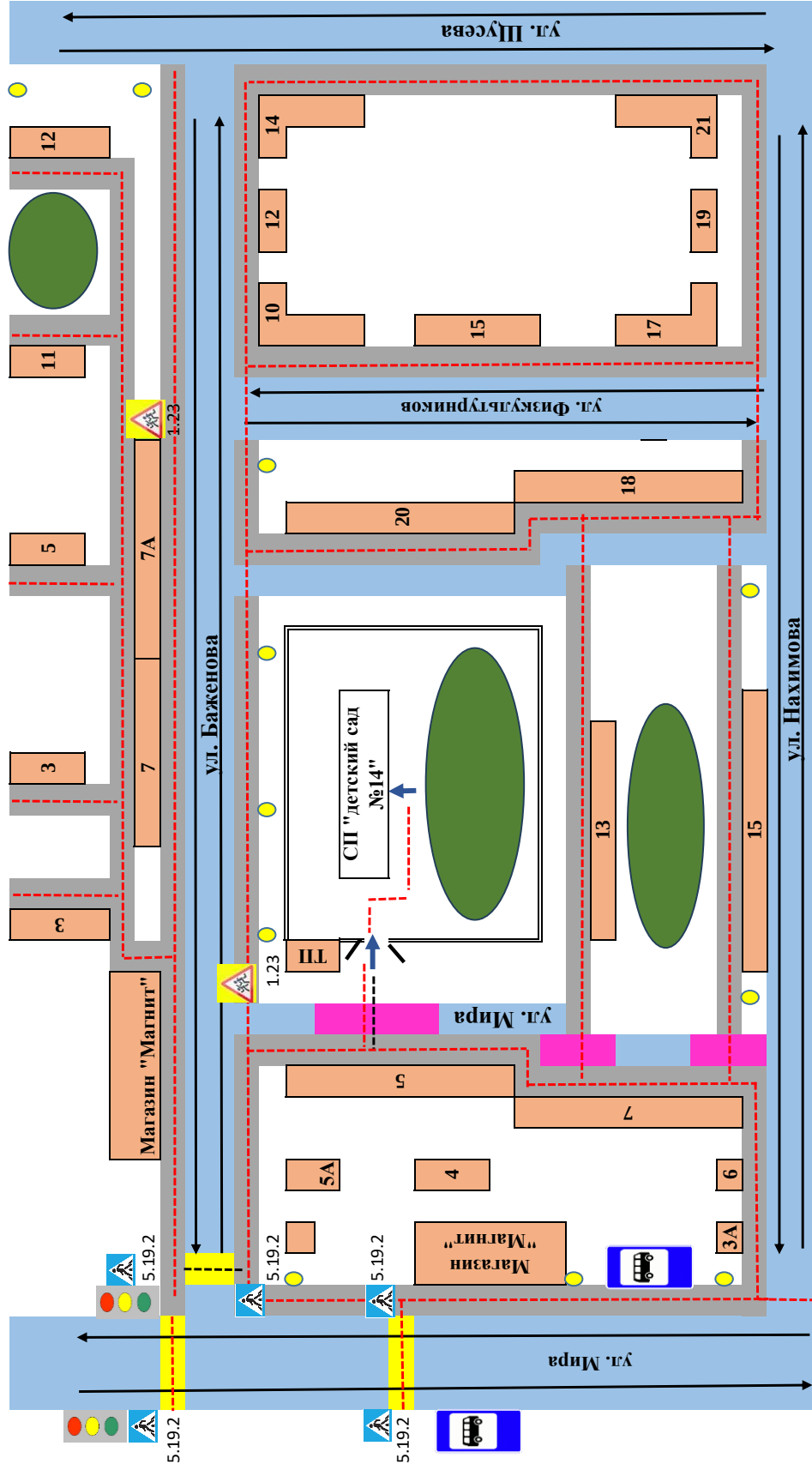
1.2.1 План – схема района расположения СП «Детский сад №14» ГБОУ ООШ №28 г.о.Сызрань пути движения транспортных средств и детей.
